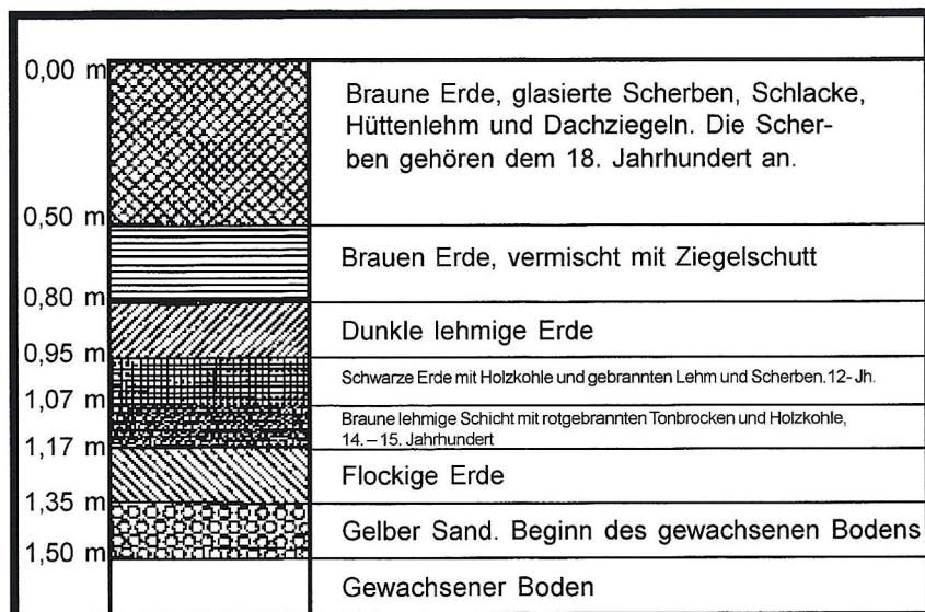
Bild 1: Ergebnis der Bohrungen von Dr. Plath im Bereich der Abtei von 1956 [nach Krause]
