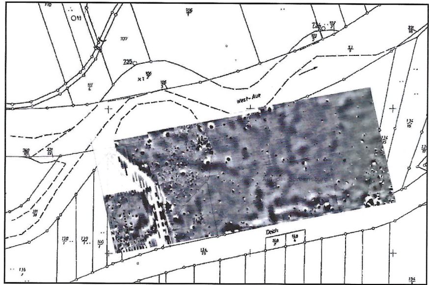
Abb. 1: Magnetometer-Survey November 2001. Das Flurstück „Burg“ zeigt Konzentrationen punktförmiger Anomalien des Erdmagnetfeldes. Im Flurstück „Spreensburg“ sind verlandete Altarme der Aue zu erkennen.
