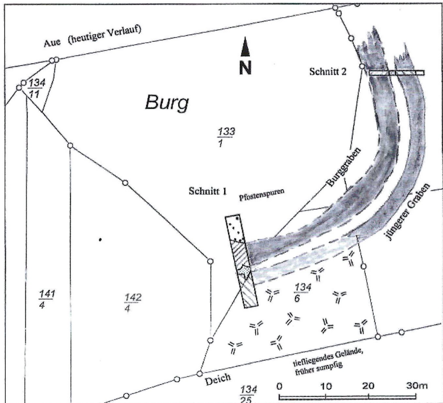
Abb.2: Katasterplan der „Burg“ mit den eingezeichneten Grabungsschnitten und den Befunden. Der Verlauf des jüngeren Grabens entspricht einem stärkeren Graswuchs im Gelände.
