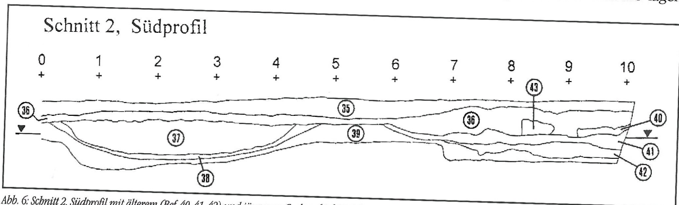
Abb. 6: Schnitt 2, Südprofil mit älterem (Bef. 40, 41, 42) und jüngerem Graben (Bef. 37, 38).
