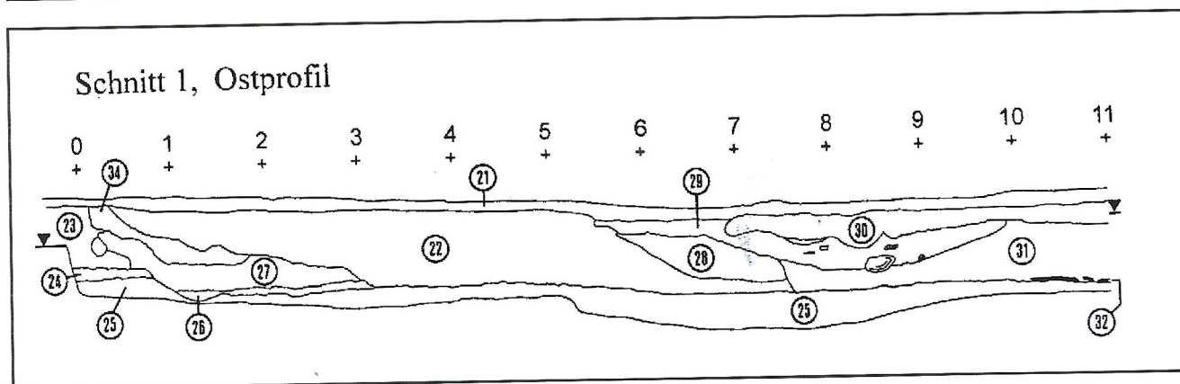
Abb. 5: Schnitt 1, Ostprofil mit mehrphasigem Grabensystem:
